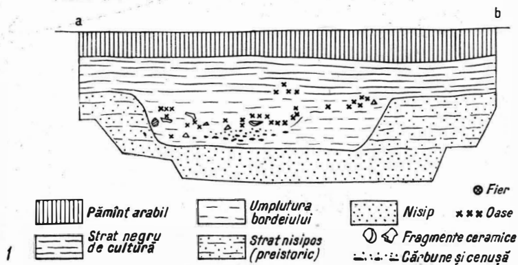
Profil a-b
